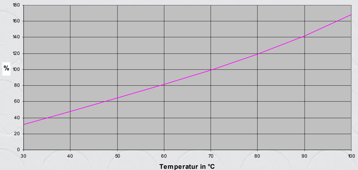
Wärmeübertragungsleistung von Heatpipes in % in Abhängigkeit von der Einspeisetemperatur T_e (Leistung bei 70^\circ\text{C} = 100\% )
